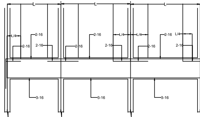
FB5/FB6/FB7/FB8/FB9(230X400) STIRRUP:8@125 C/C
