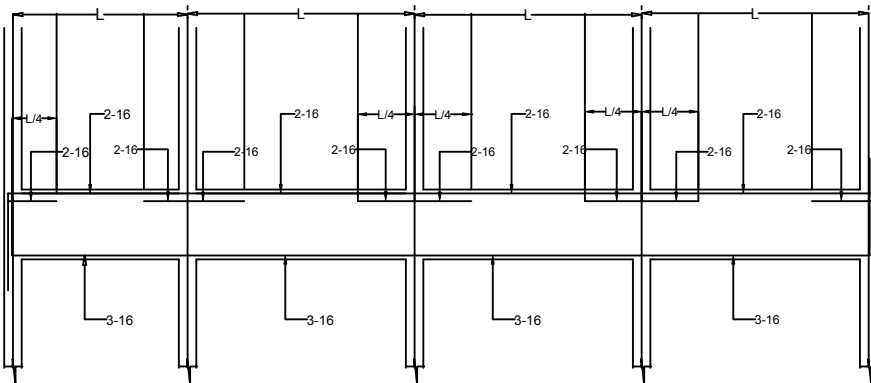
FB1/FB2/FB3/FB4(230X400) STIRRUP:8@125 C/C
